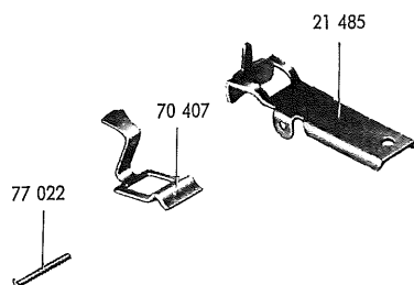
Fig. 9a Kupplung, zerlegt
