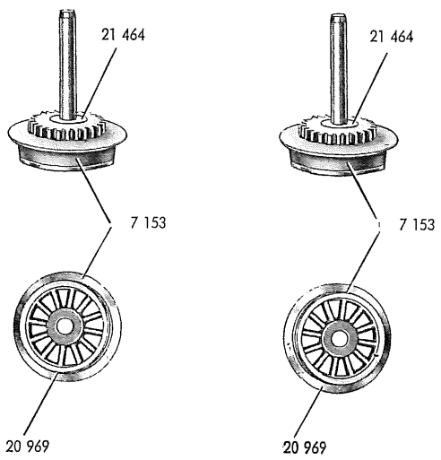
Fig. 5 Treibachsteil und Treibrad
