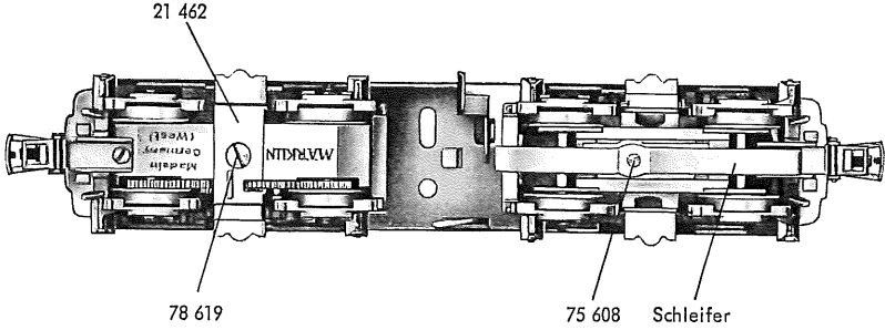
Fig. 3 Motordrehgestell
