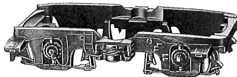
Fig. 8 Drehgestellrahmen
