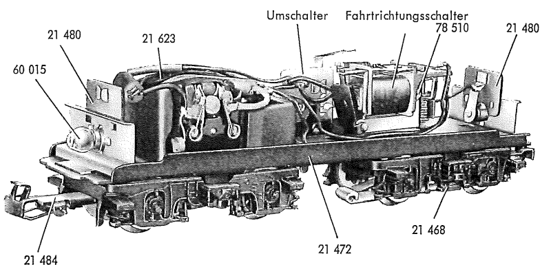
Fig. 2 Fahrgestell
