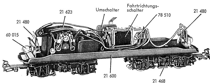
Fig. 2 Fahrgestell
