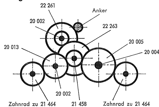
Fig. 5 Treibachsenteil und Treibrad
