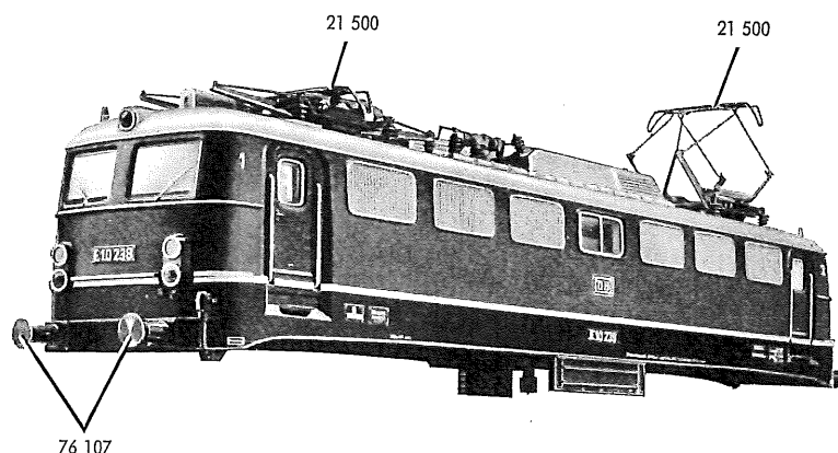
Fig. 1 Lokomotiv-Aufbau
