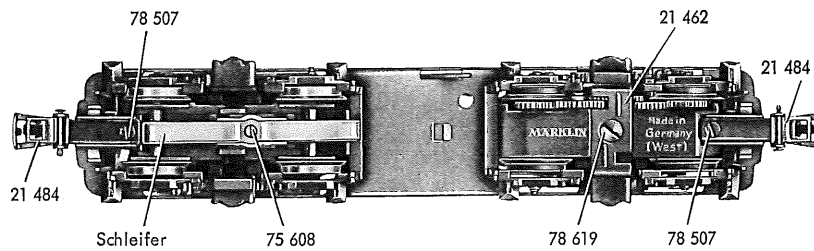
Fig. 3 Motordrehgestell
