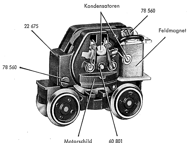
Fig. 3 Motordrehgestell
