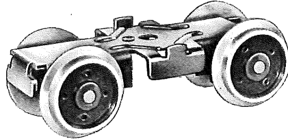
Fig. 7 Drehgestellrahmen (Treibgestell)
