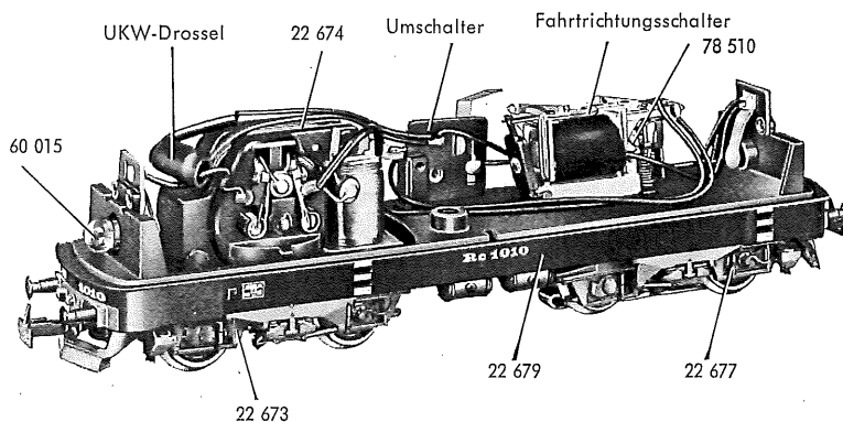
Fig. 2 Fahrgestell
