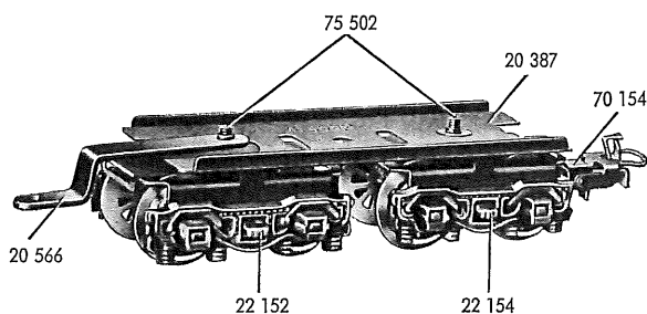
Fig. 2a Vorderes Drehgestell (von unten gesehen)
