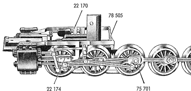
Fig. 7 Laufgestell
