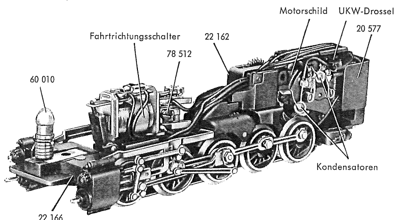
Fig. 2 Fahrgestell
