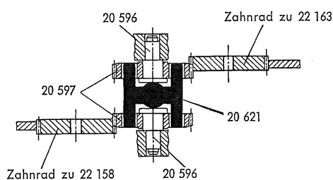
Fig. 4a Getriebekupplung
