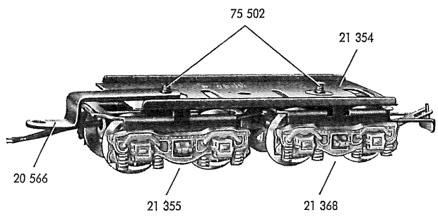
Fig. 2 Fahrgestell
