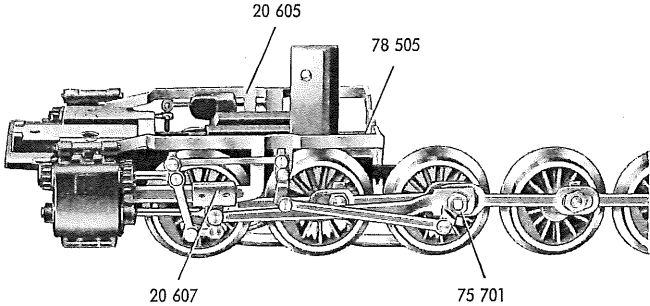
Fig. 7 Laufgestell
