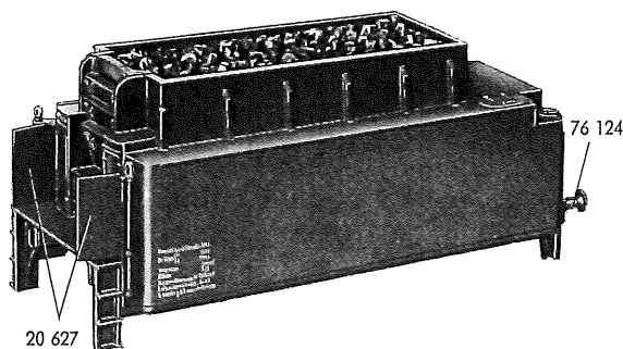
Fig. 1 Tender-Aufbau
