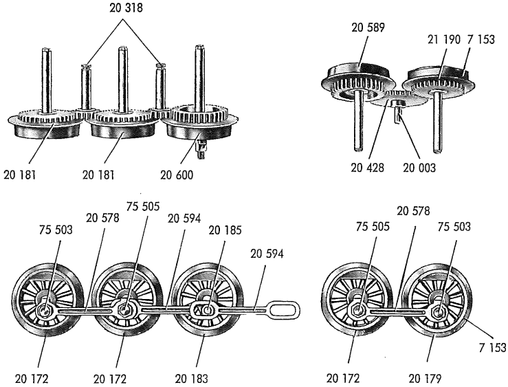
Fig. 6 Gestänge
