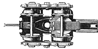
Fig. 2b Hinteres Drehgestell (von unten gesehen)
