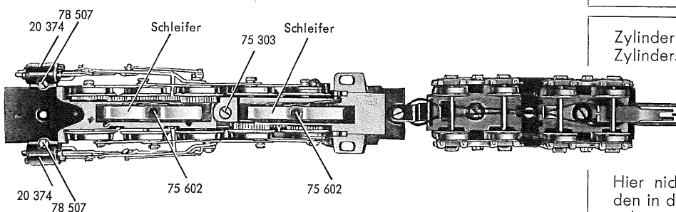
Fig. 2a Fahrgestelle (von unten gesehen) Lokomotive ohne Laufgestell
