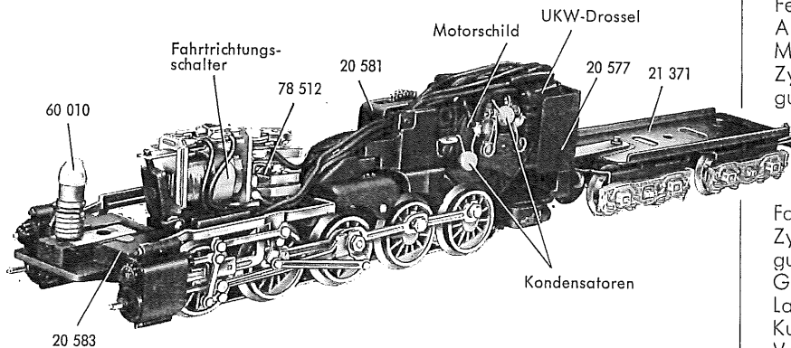
Fig. 2 Fahrgestell mit Tenderfahrgestell
