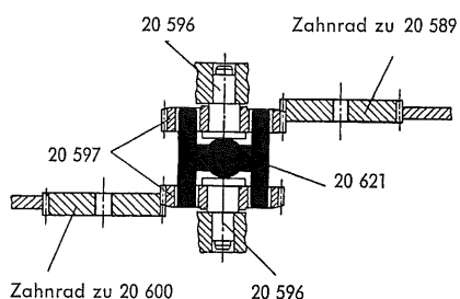
Fig. 4a Getriebekupplung
