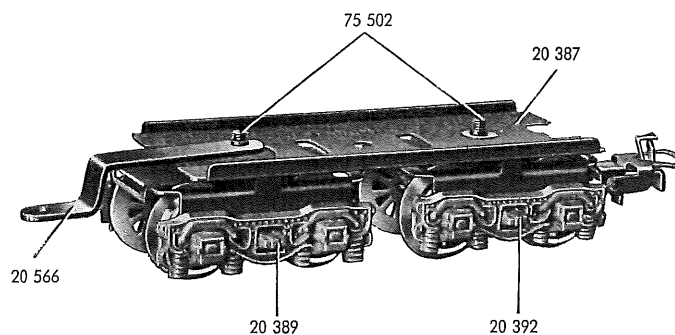
Fig. 2 Fahrgestell
