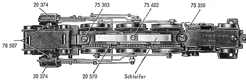
Fig. 3 Treibgestell
