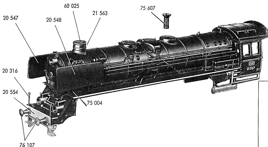
Fig. 1 Lokomotiv-Aufbau
