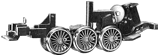
Fig. 4 Anordnung der Getrieberäder
