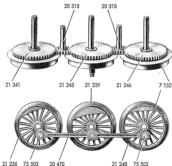
Fig. 5 Treibachsenteile und Treibräder
