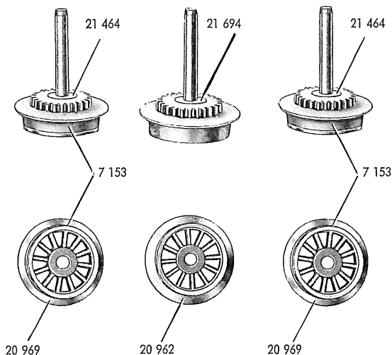
Fig. 5 Treibachsenteile und Treibräder
