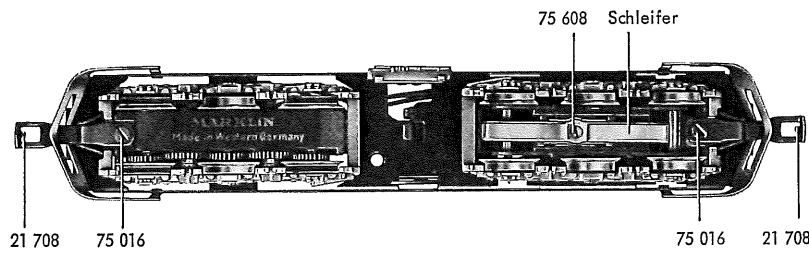
Fig. 3 Motordrehgestell
