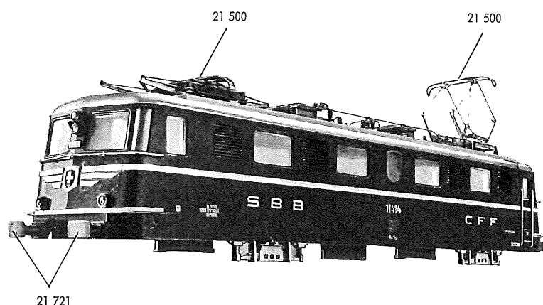
Fig. 1 Lokomotiv-Aufbau mit Scherenstromabnehmern
