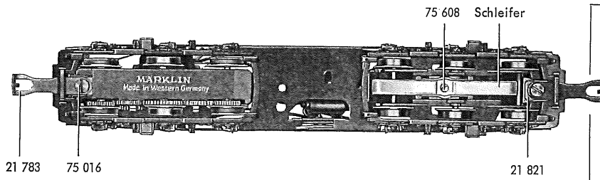
Fig. 3 Motordrehgestell
