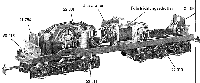
Fig. 2 Fahrgestell
