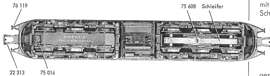
Fig. 2b Fahrgestell (von unten gesehen)
