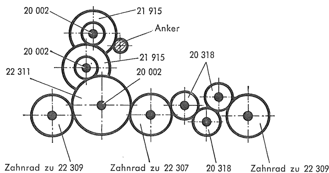
Fig. 5 Treibachseile und Treibräder
