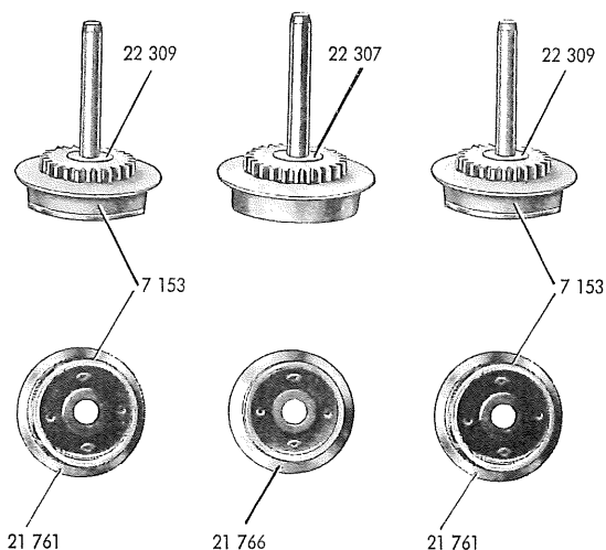
Fig. 5 Treibachseile und Treibräder
