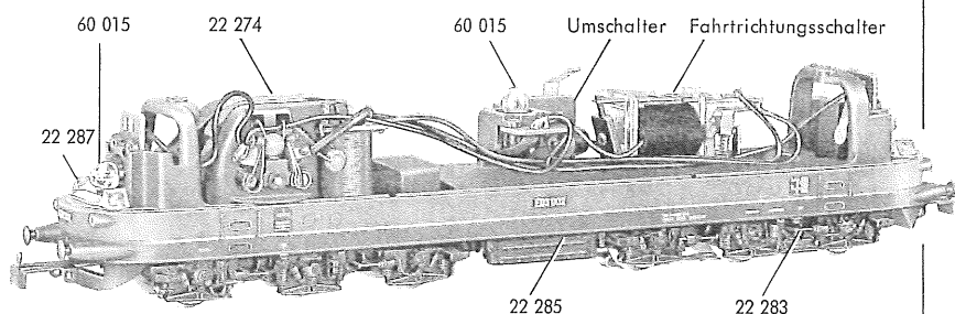
Fig. 2 Fahrgestell
