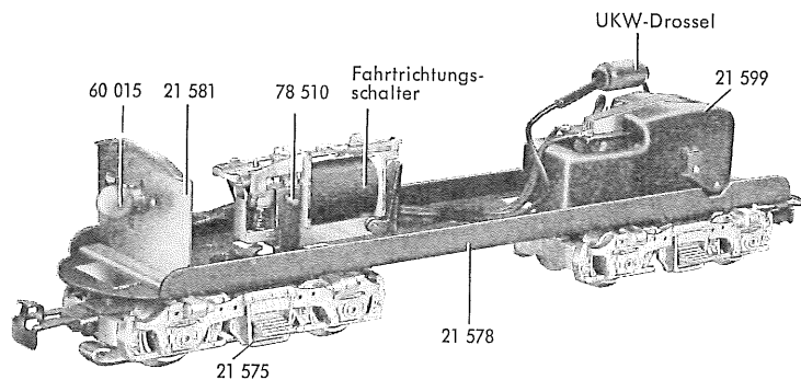
Fig. 2 Fahrgestell
