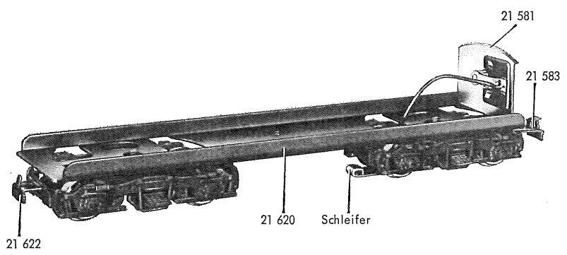
Fig. 9 Fahrgestell
