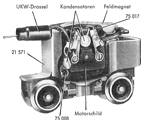
Fig. 3 Motordrehgestell
