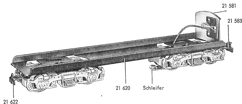
Fig. 9 Fahrgestell
