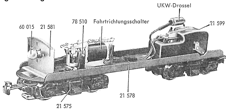
Fig. 2 Fahrgestell
