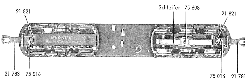
Fig. 2a Fahrgestell (von unten gesehen)
