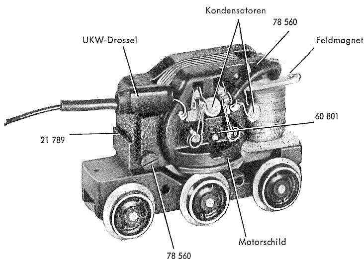
Fig. 3 Motordrehgestell
