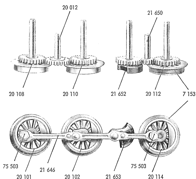
Fig. 5 Treibachsenteile und Treibräder
