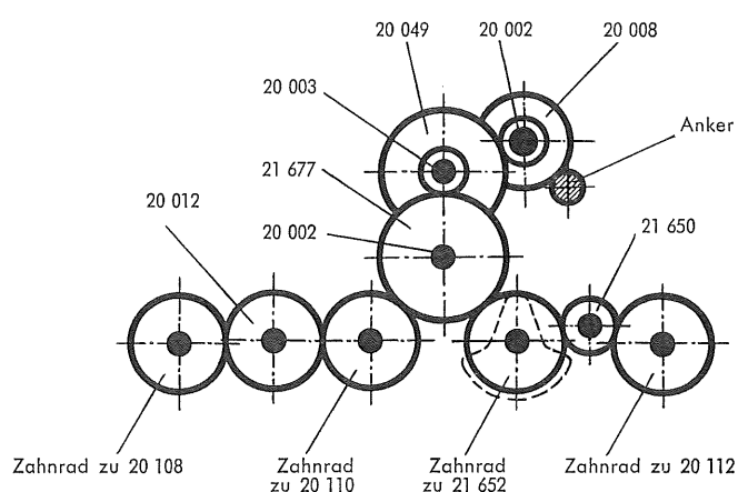
Fig. 5 Treibachsenteile und Treibräder
