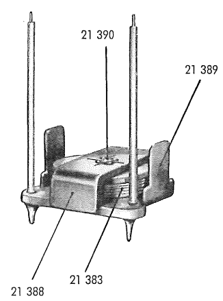
Fig. 7a Magnet zur TELEX-KUPPLUNG
