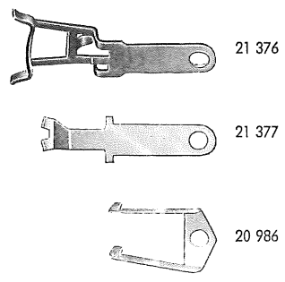
Fig. 7 MÄRKLIN-TELEX-KUPPLUNG
