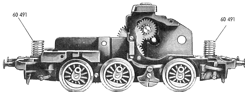
Fig. 4 Anordnung der Getrieberäder
