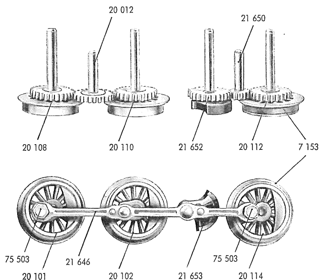
Fig. 5 Treibachsenteile und Treibräder
