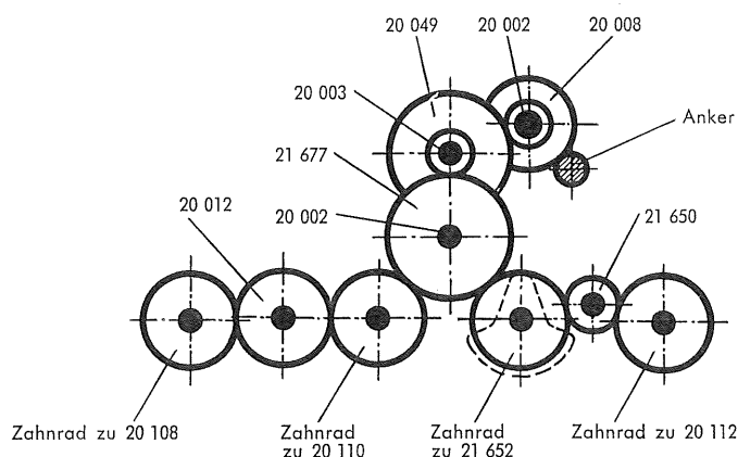
Fig. 4 Anordnung der Getrieberäder
