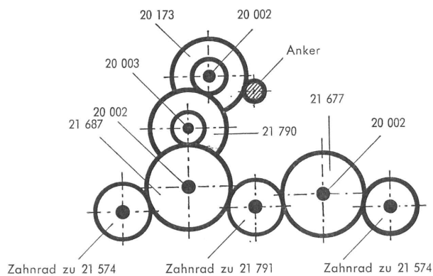
Fig. 5 Treibachseile und Treibräder
