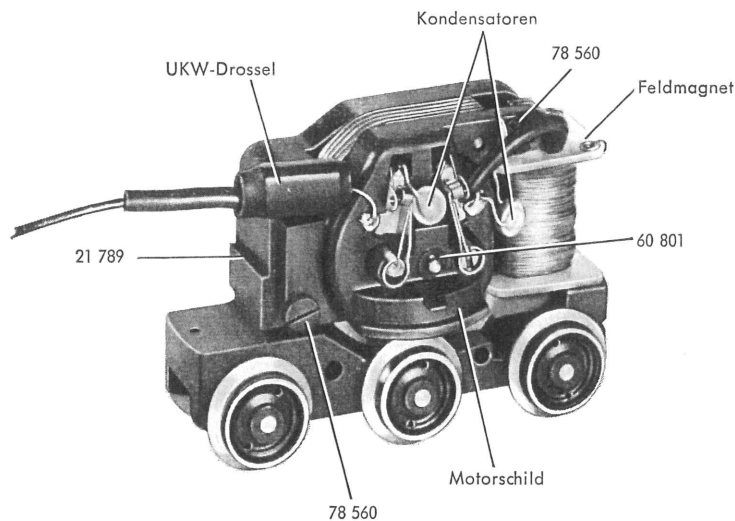
Fig. 3 Motordrehgestell
