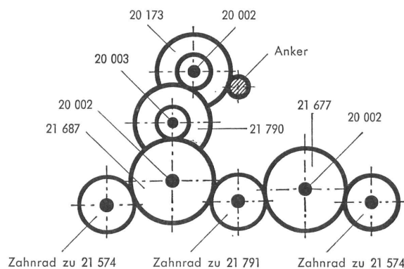
Fig. 5 Treibachsenteil und Treibrad
