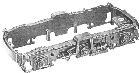
Fig. 8 Drehgestellrahmen
