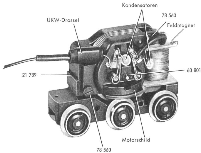
Fig. 3 Motordrehgestell
