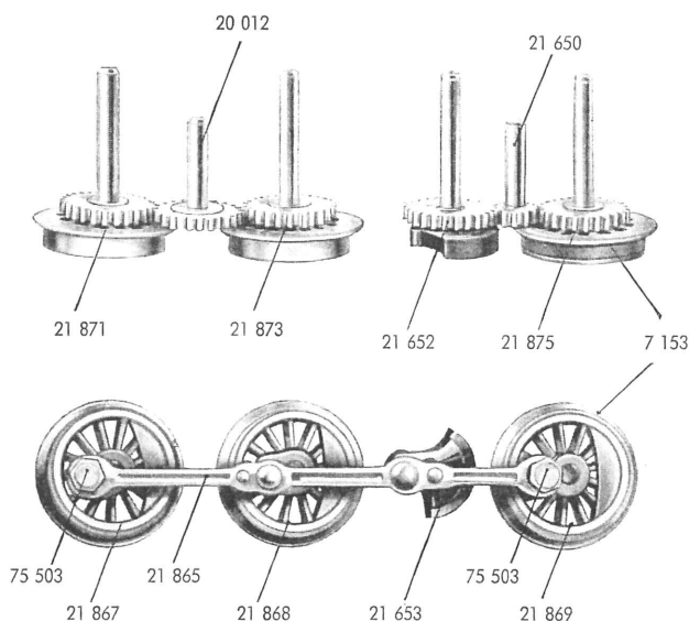
Fig. 5 Treibachsenteile und Treibräder
