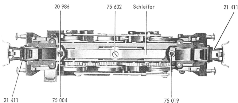
Fig. 2a Fahrgestell (von unten gesehen)
