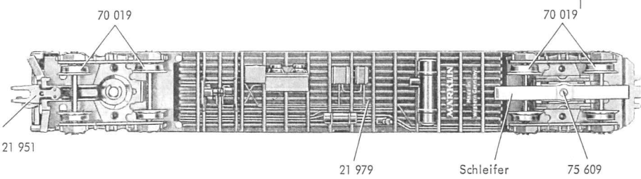
Fig. 12a Fahrgestell (von unten gesehen)
