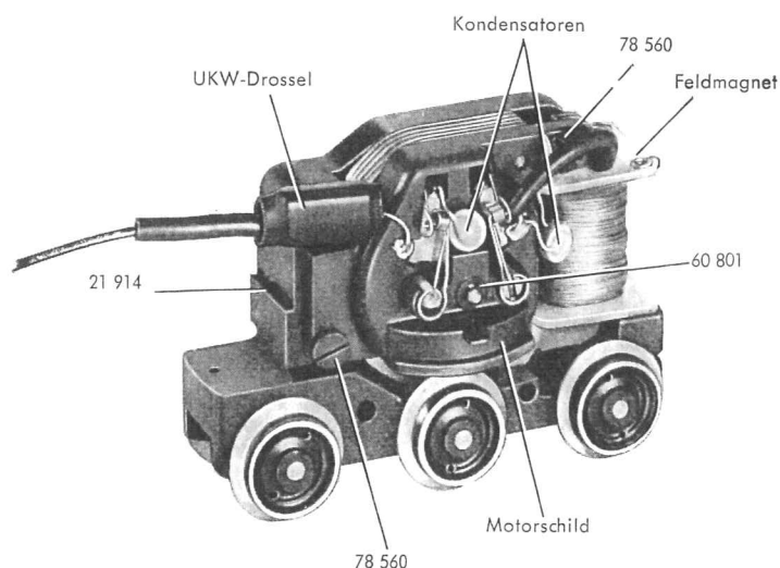
Fig. 3 Motordrehgestell
