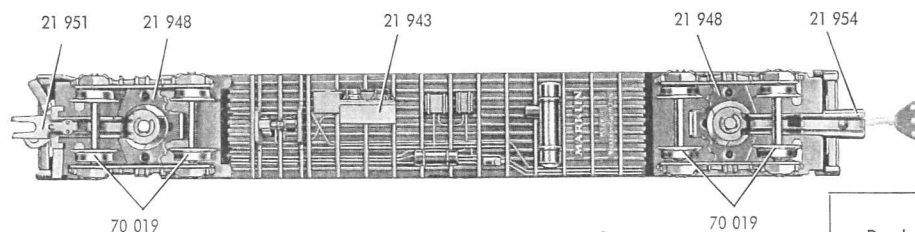
Fig. 10a Fahrgestell (von unten gesehen)
