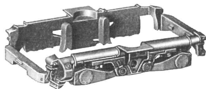
Fig. 8 Drehgestellrahmen (Treibgestell)
