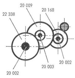
Fig. 4 Anordnung der Getrieberäder
