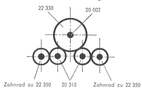
Fig. 7 Treibachsenteile und Treibräder
