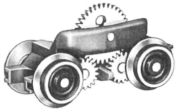
Fig. 6 Anordnung der Getrieberäder im Treibgestell
