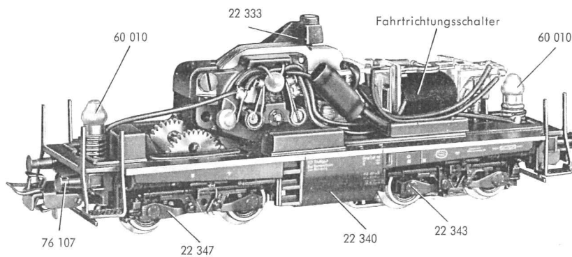
Fig. 2 Fahrgestell
