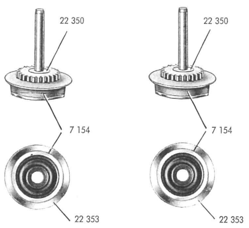
Fig. 7 Treibachsenteile und Treibräder
