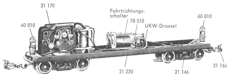
Fig. 3 Fahrgestell
