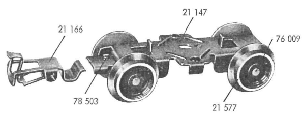
Fig. 8 Drehgestellrahmen (zum Getriebemotor)
