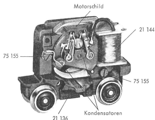
Fig. 4 Getriebemotor
