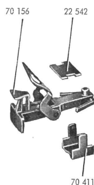
Fig. 7 Drehgestellrahmen (Drehgestell) Kupplung
