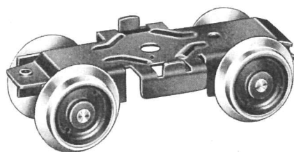
Fig. 7 Drehgestellrahmen (Drehgestell) Kupplung
