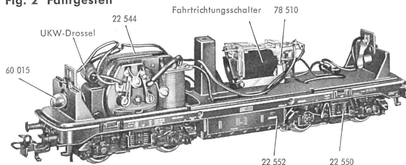
Fig. 2 Fahrgestell
