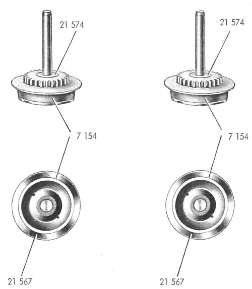
Fig. 5 Treibachsenteil und Treibrad
