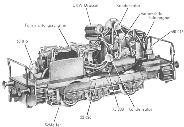
Fig. 2 Fahrgestell
