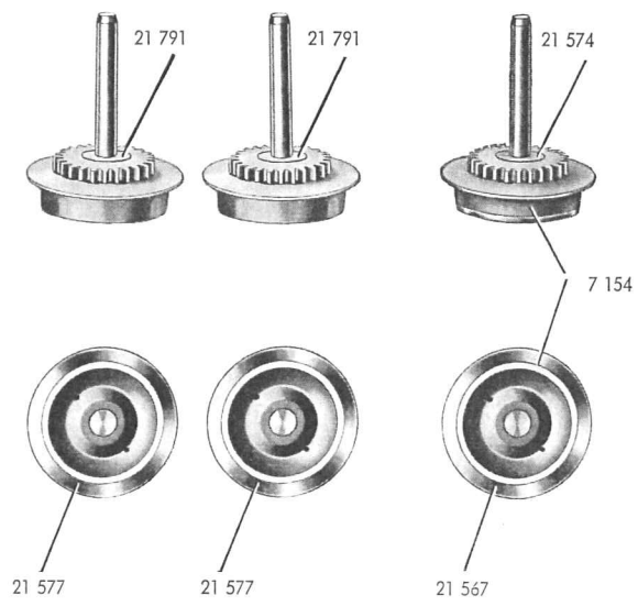
Fig. 5 Treibachsenteile und Treibräder
