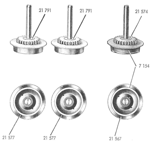
Fig. 5 Treibachsenteile und Treibräder
