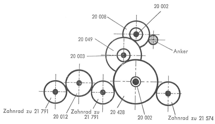
Fig. 5 Treibachsenteile und Treibräder
