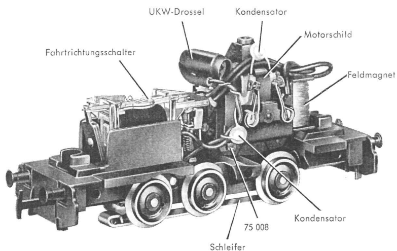
Fig. 2 Fahrgestell
