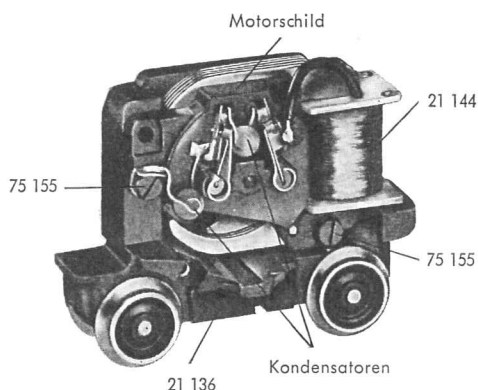
Fig. 4a Drehgestellrahmen
