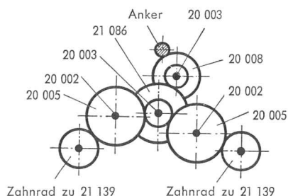
Fig. 6 Treibachsenteil und Treibrad
