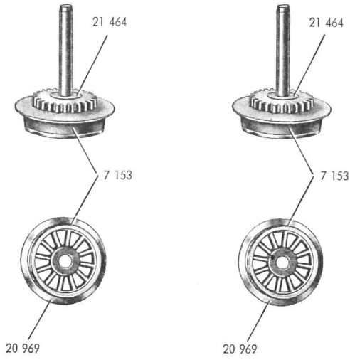
Fig. 6 Treibachsenteil und Treibrad
