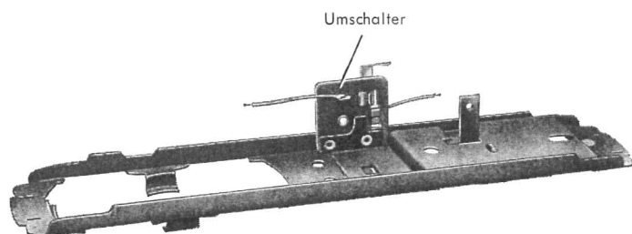
Fig. 2 Rahmen mit Umschalter
