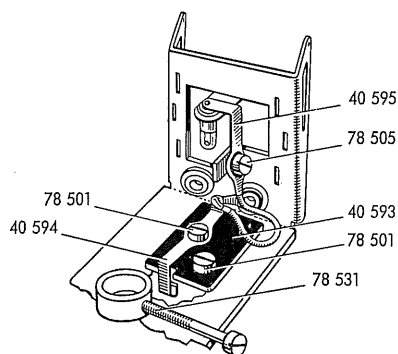
Fig. 1a Kranhaussockel
