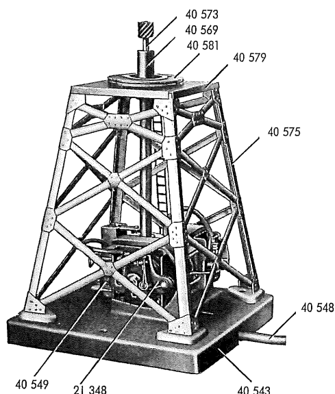
Fig. 4 Antrieb der Hauptwelle
