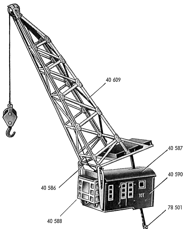
Fig. 1a Kranhaussockel
