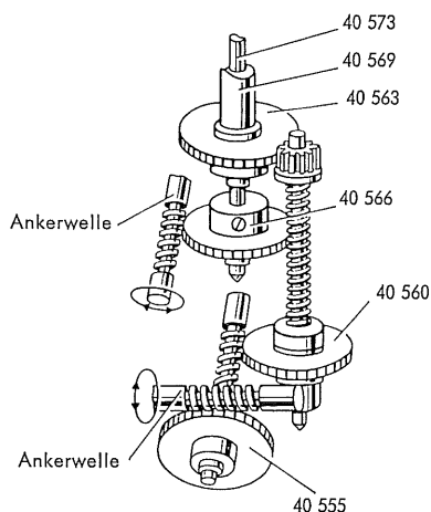
Fig. 4 Antrieb der Hauptwelle
