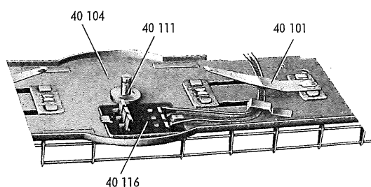
Fig. 1b Drehbühne von unten gesehen (Teilansicht)
