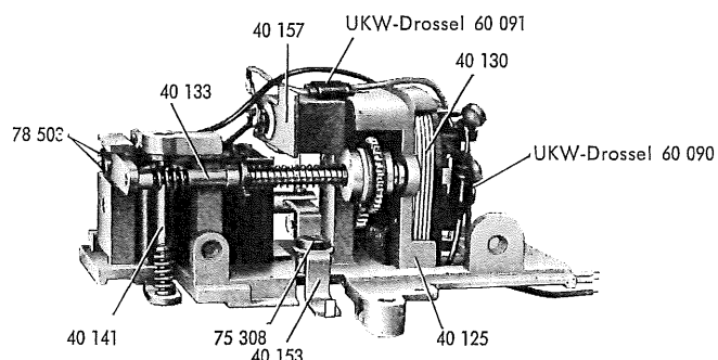
Fig. 2 Drehscheibenantrieb
