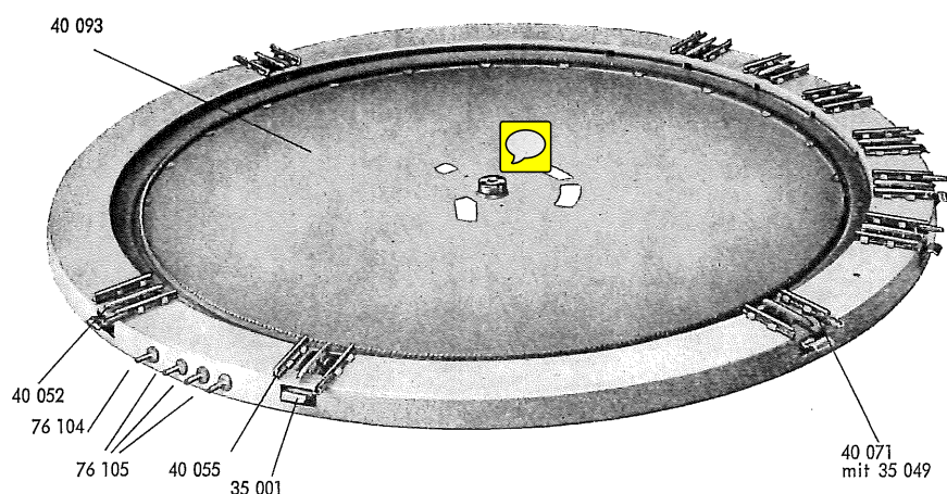
Fig. 1 Drehgrube
