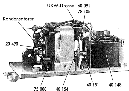
Fig. 3 Drehscheibenantrieb (Magnetseite)
