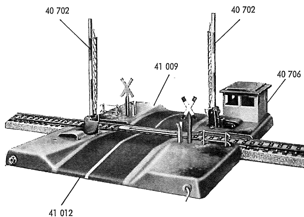
Fig. 1 Bahnübergang, eingleisig
