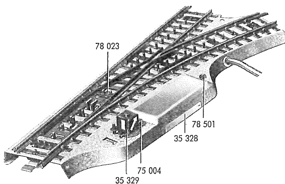
Fig. 1 Rechtsweiche für elektromagnetischen Betrieb
