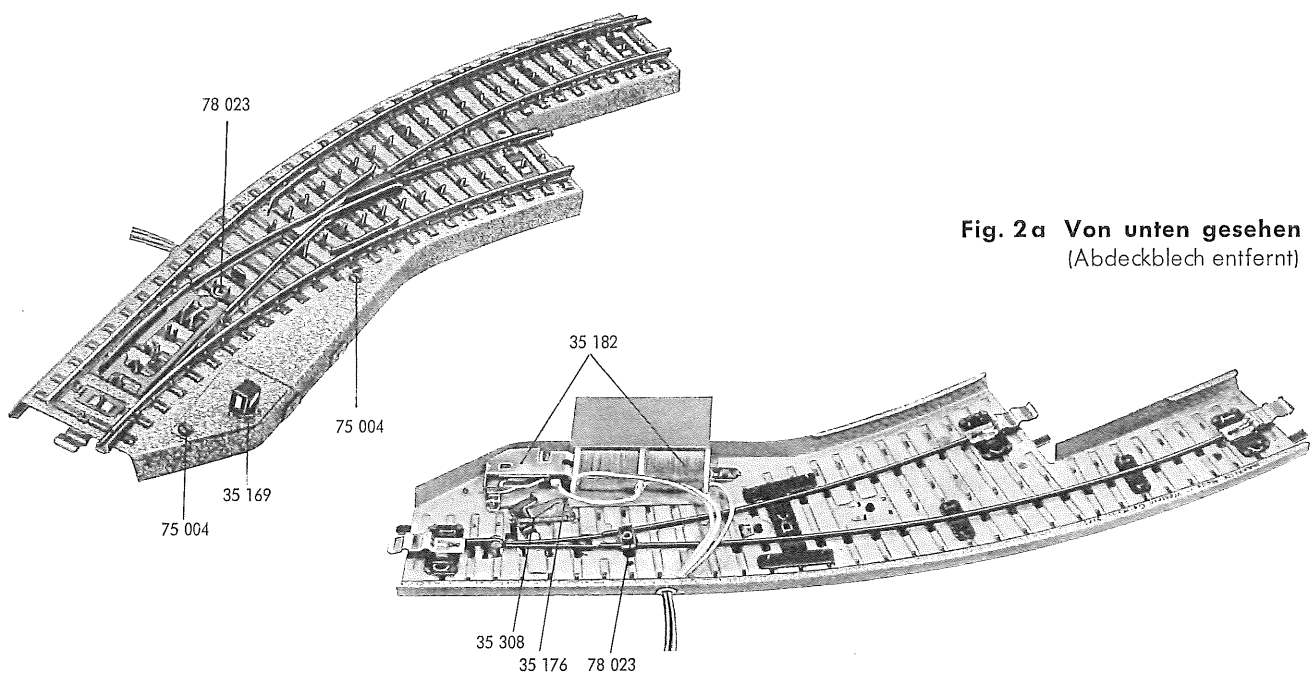
Fig. 2 Rechtsweiche für elektromagnetischen Betrieb
