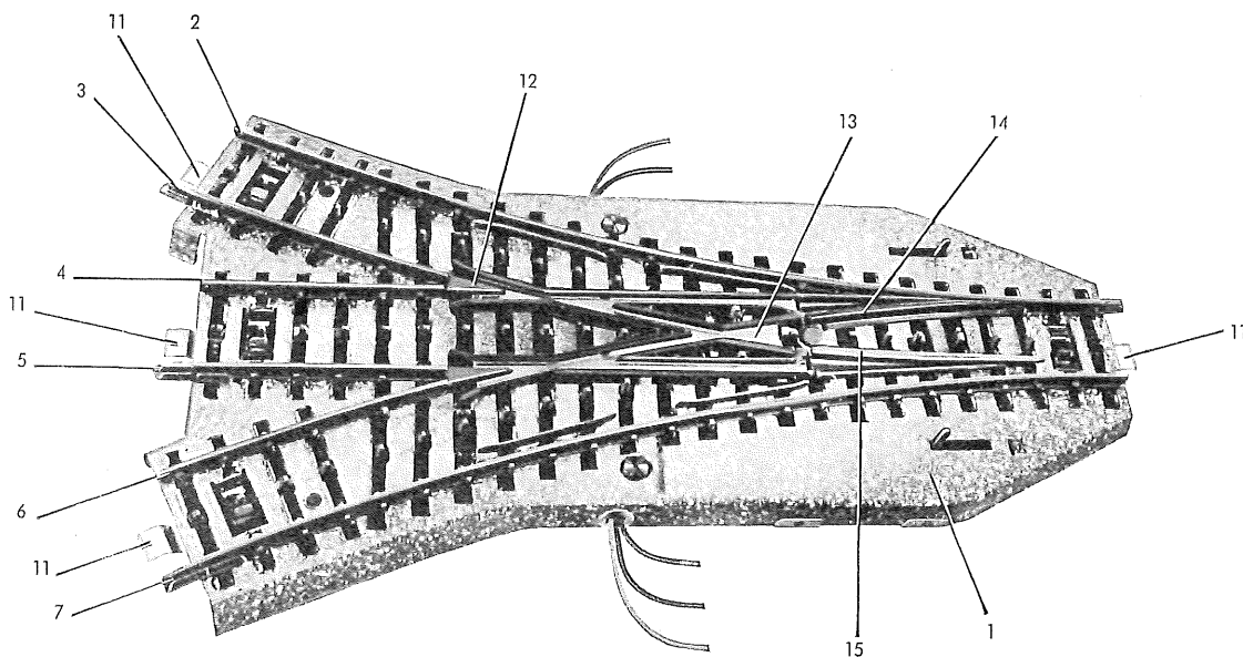
Fig. 1 Weichenoberteil (von oben gesehen)
